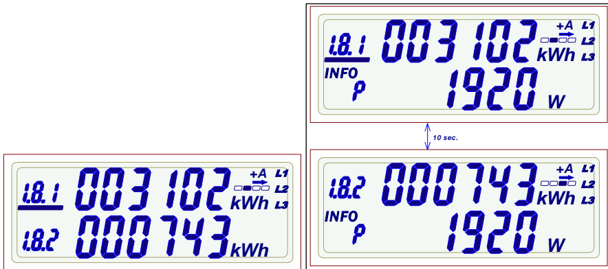
Abb. 10: Doppeltarif-Bezugszähler ohne (links) und mit (rechts) Leistungsanzeige
